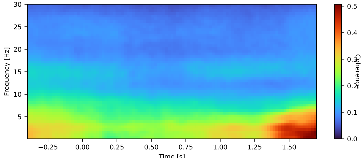
8B (0) - dPFC (6)
